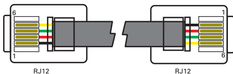
kabllloja e lidhjes RJ12 mes EM44 dhe EM49 / connection cable RJ12 between EM44 and EM49
