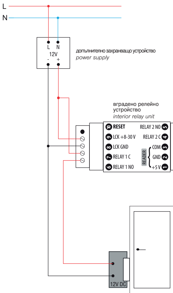
електрическа ключалка electric lock
